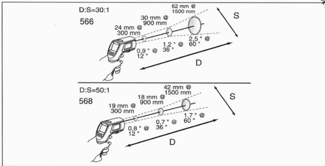
Figure 5. Distância e tamanho do ponto focal
