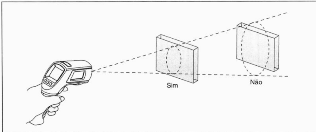
Figura 6. Campo de visão
