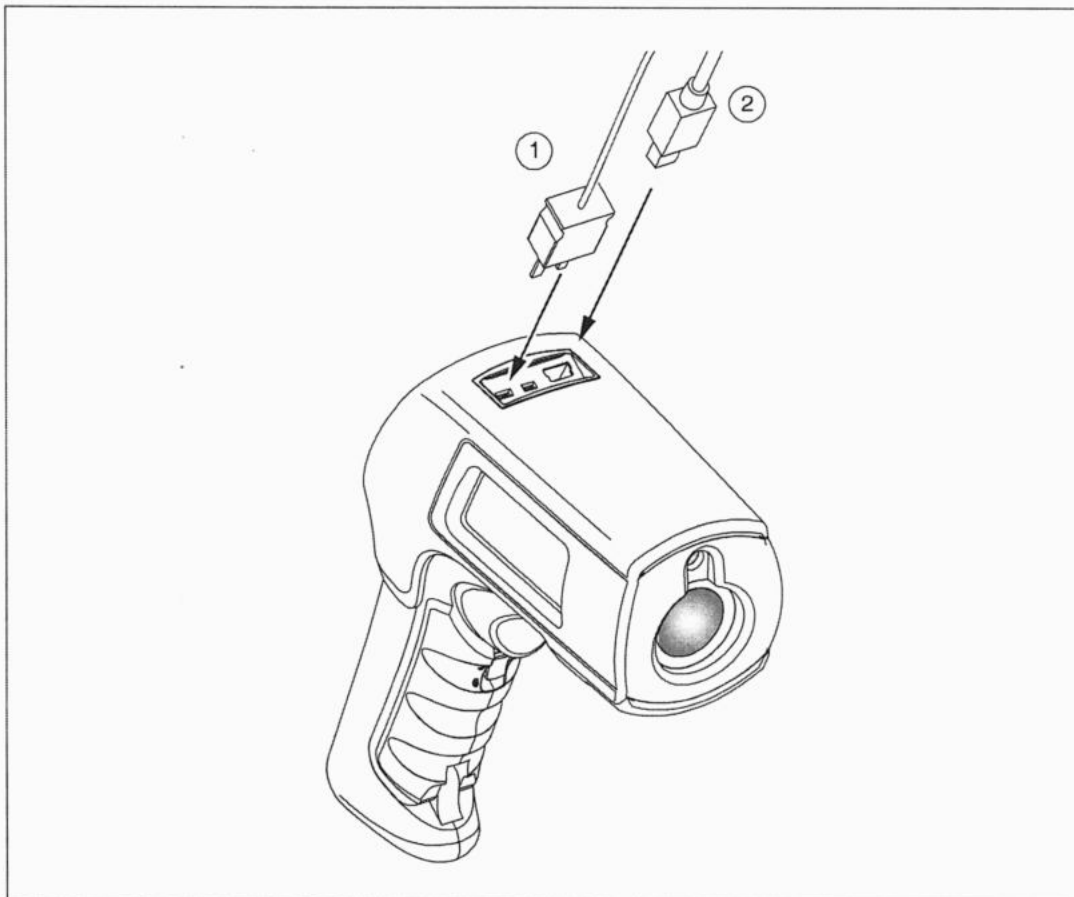
Figura 7. Conexões de termopar e USB
