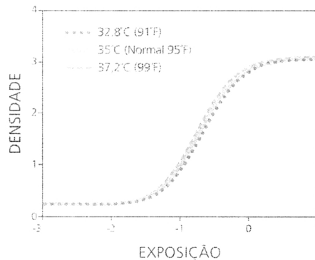
Efeito do filme MXG de temperatura com ecrans regulares LANEX
