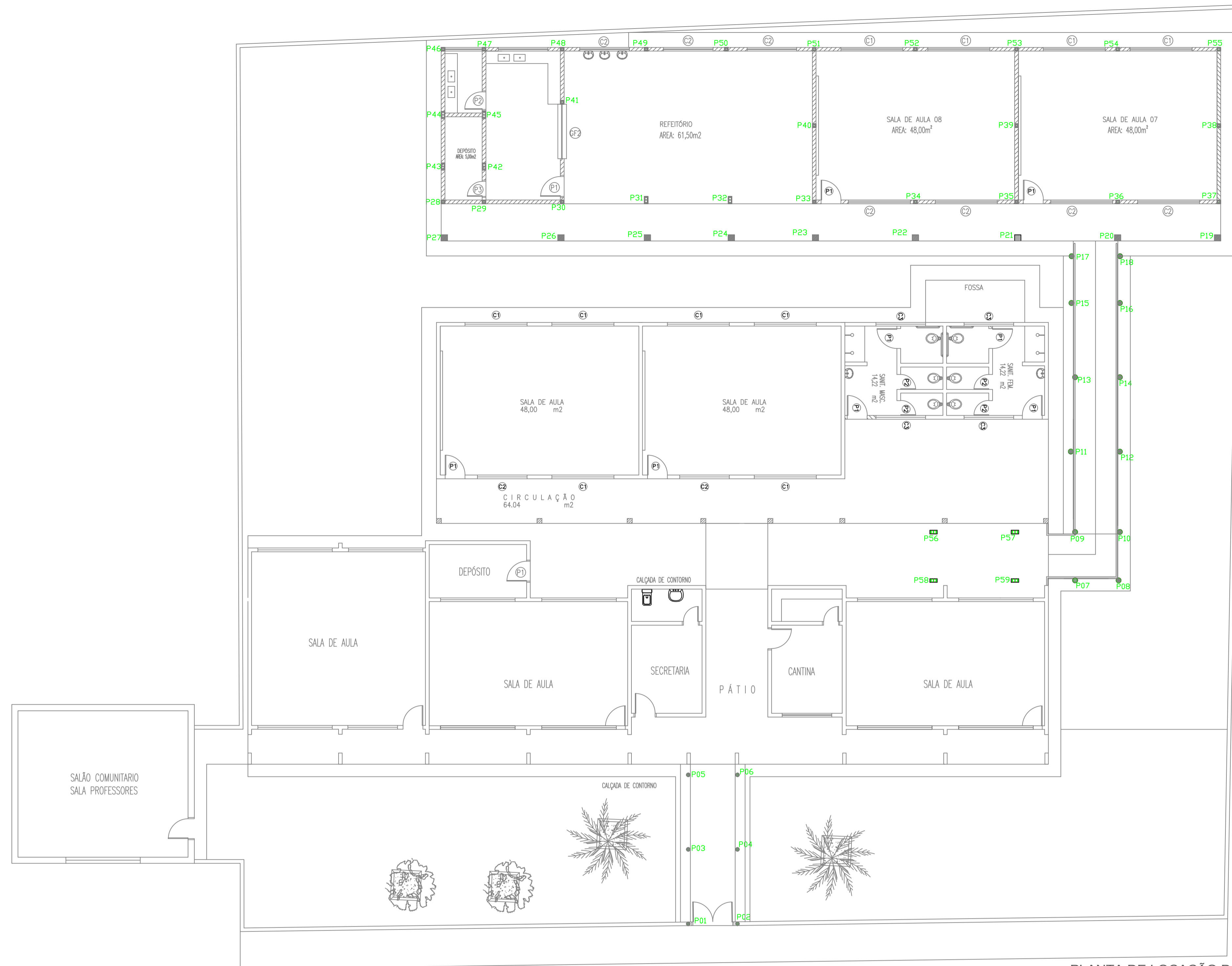
12 PLANTA DE LOCAÇÃO DOS PILARES ESC.: 1/100
