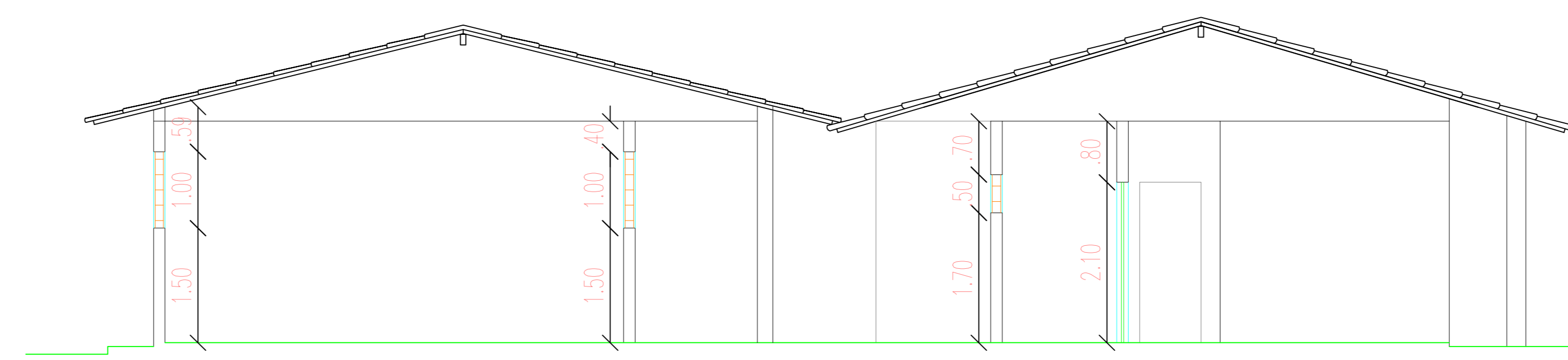
5 CORTE A-A ESC.: 1/75
