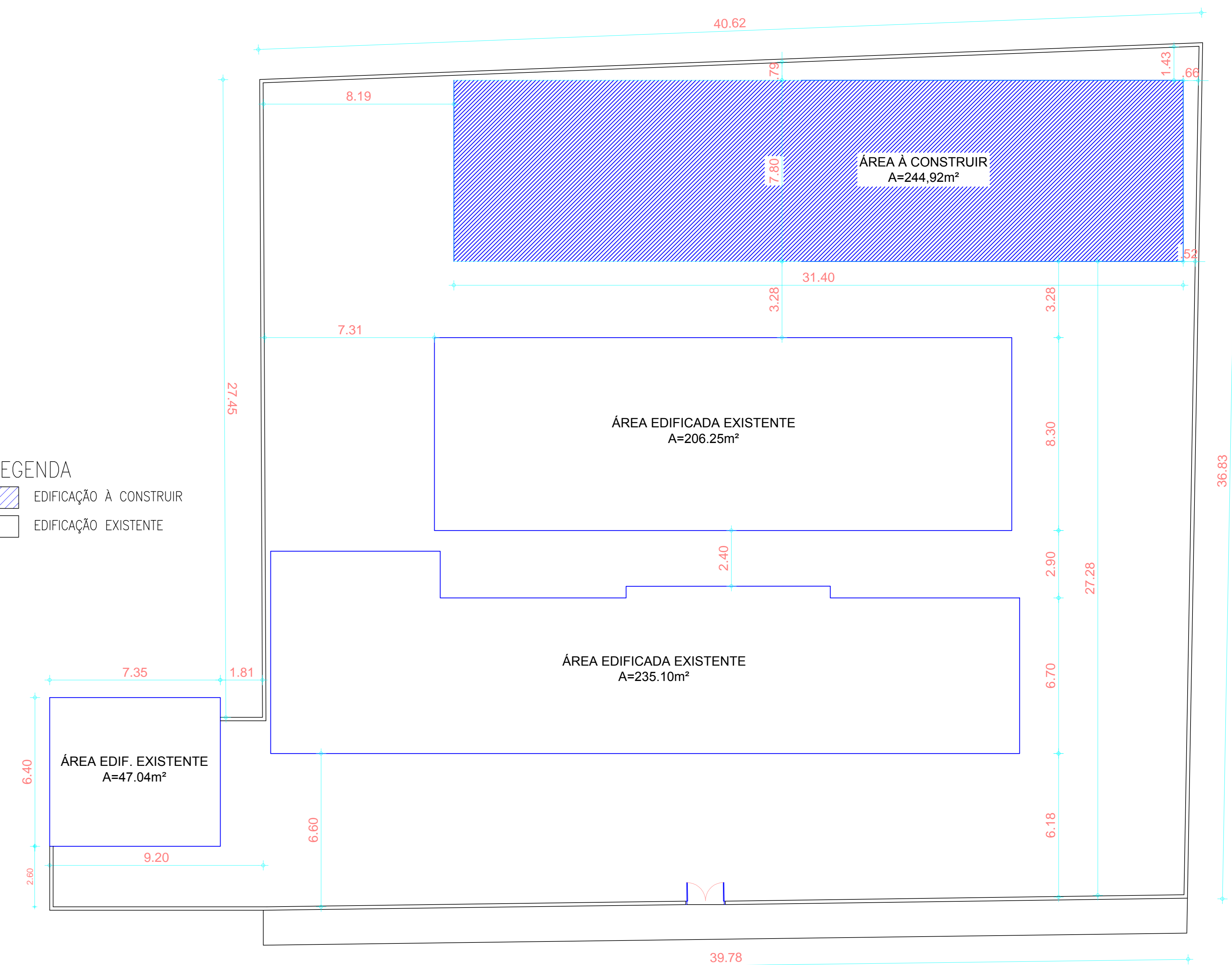
4 PLANTA SITUAÇÃO ESC.: 1/150
