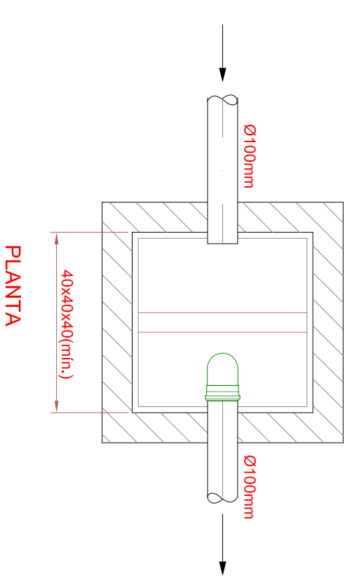
CAIXA DE GORDURA - CG ESCALA
