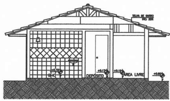
2 CORTE AA ESC.: 1/75
