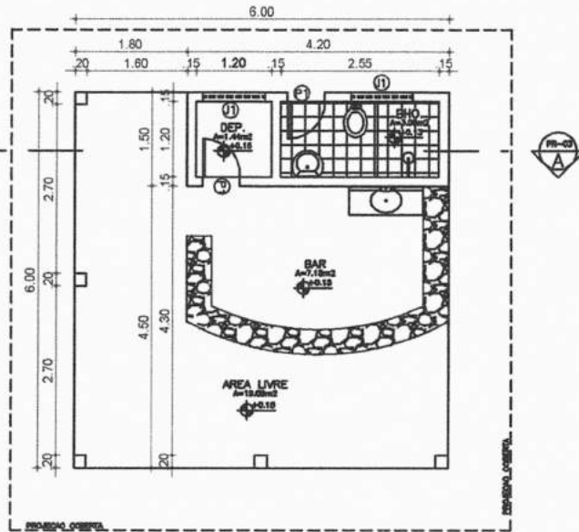
1 PLANTA BAIXA ESC.: 1/75
