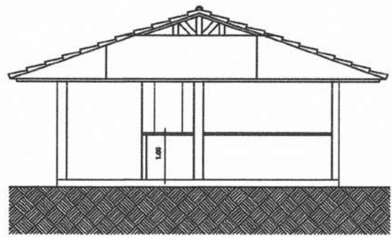
3 FACHADA ESC.: 1/75
