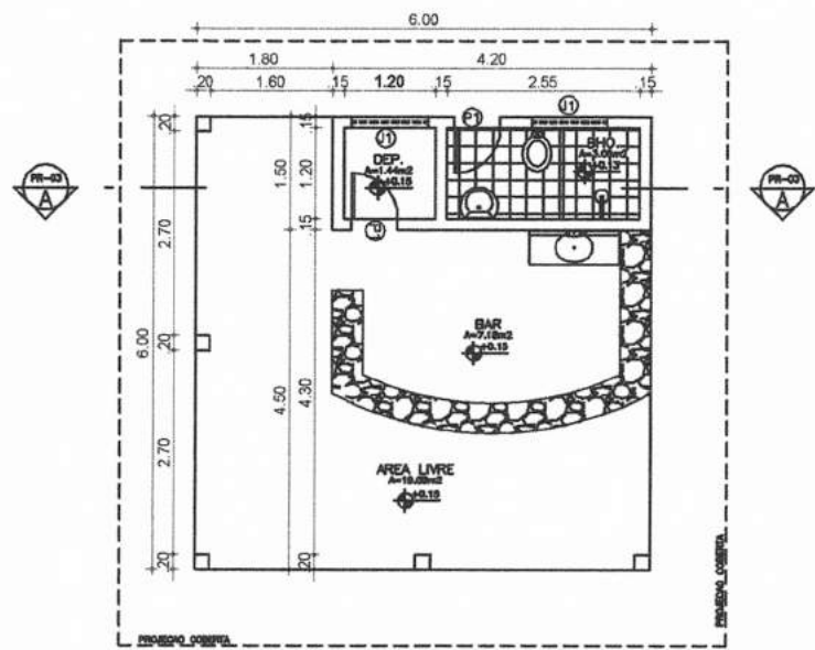
1 PLANTA BAIXA ESC.: 1/75
