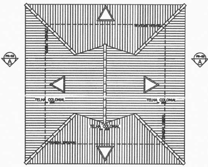
4 COBERTA ESC.: 1/75
