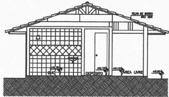
2 CORTE AA ESC.: 1/75
