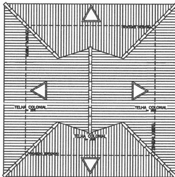
4 COBERTA ESC.: 1/75
