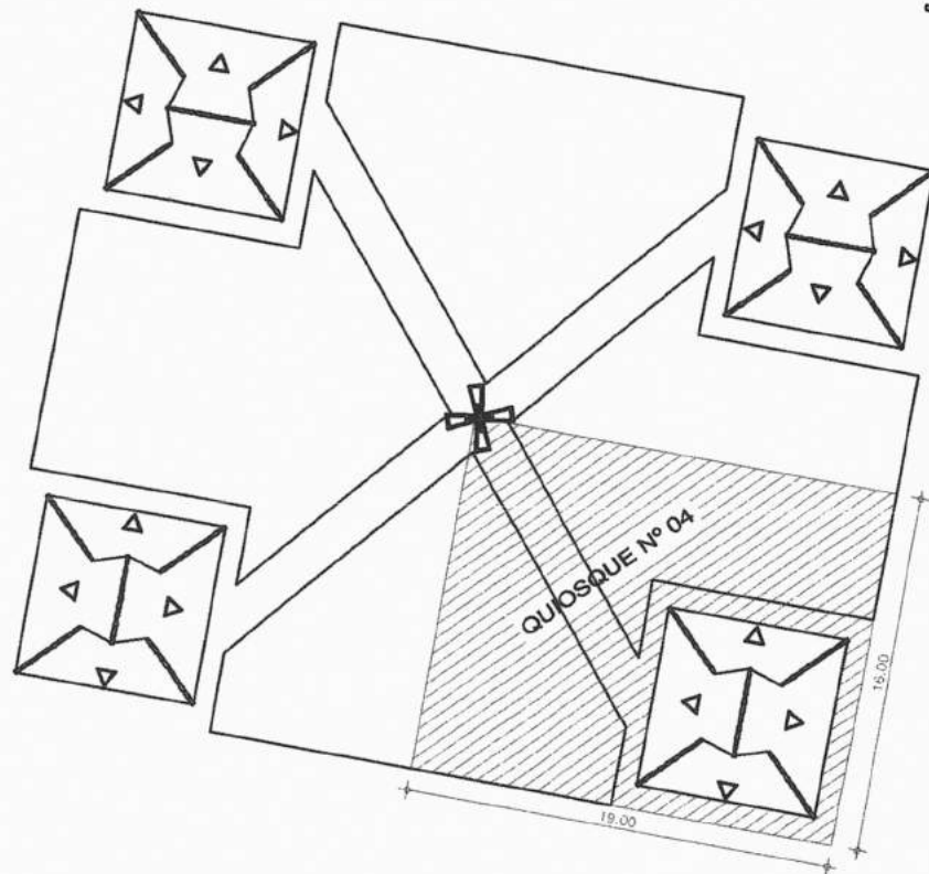
1 PLANTA SITUAÇÃO ESC.: 1/200
