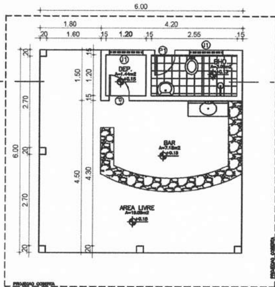
1 PLANTA BAIXA ESC.: 1/75
