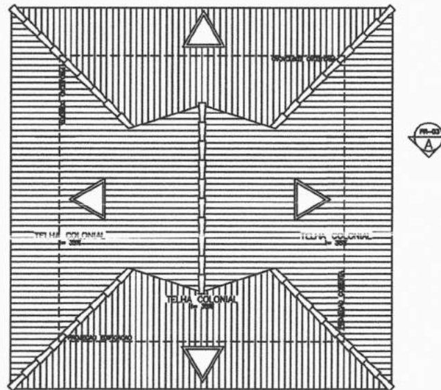
4 COBERTA ESC.: 1/75
