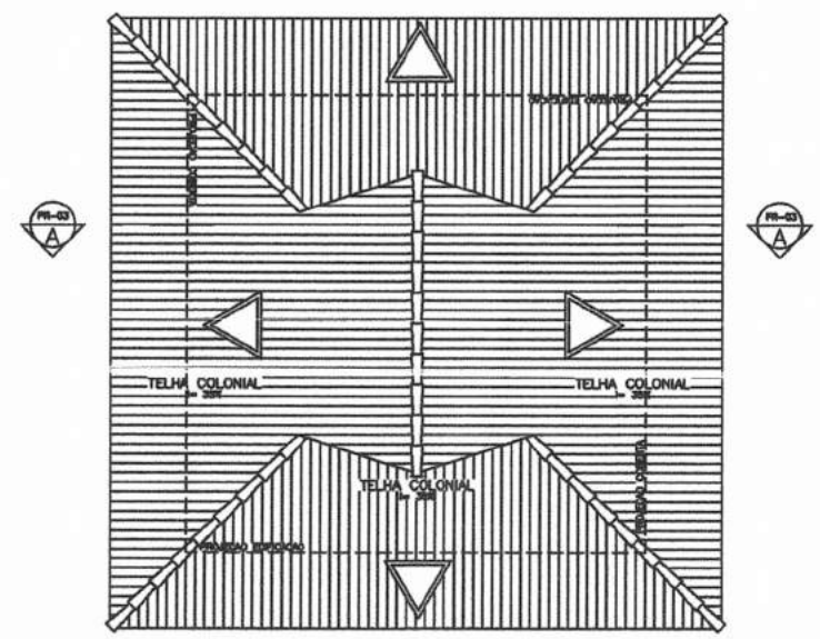
4 COBERTA ESC.: 1/75
