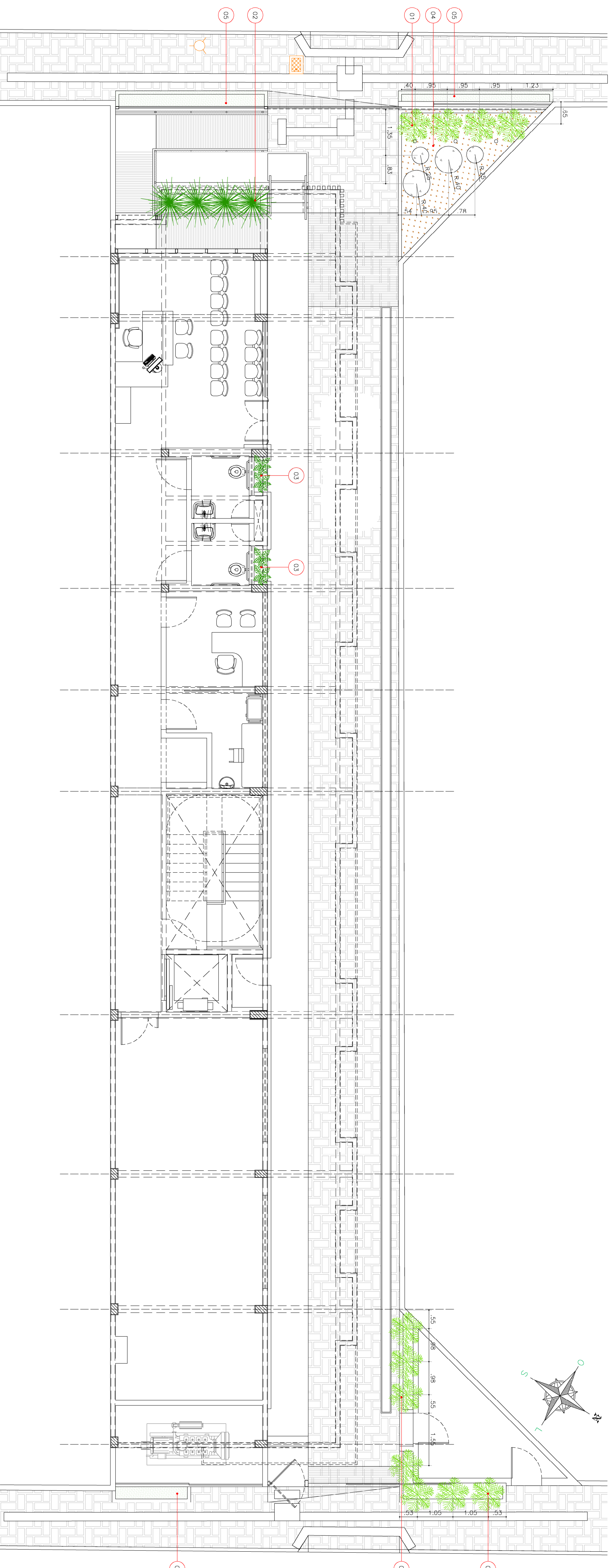
PLANTA BAIXA - TERREO
